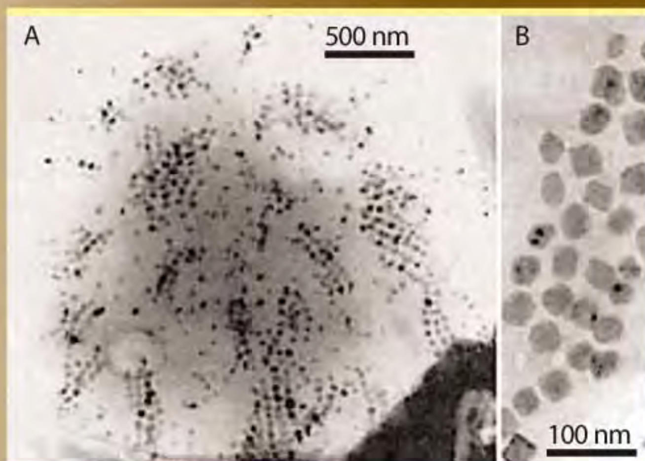
Una colonia di Magnetobatteri vista al microscopio elettronico a due diversi ingrandimenti. Sebbene le singole cellule non siano visibili, sono invece immediatamente evidenti le catene di microcristalli ferrici associati alla membrana cellulare (detti magnetosomi), che consentono a questi organismi di muoversi lungo le linee del campo magnetico terrestre, una capacità denominata magnetotassi.
