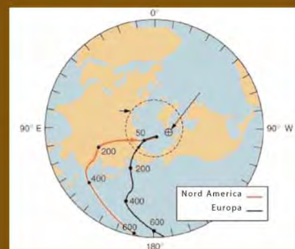
PERCORSO APPARENTE DEL POLO NORD MAGNETICO NEGLI ULTIMI 600 MILIONI DI ANNI.
