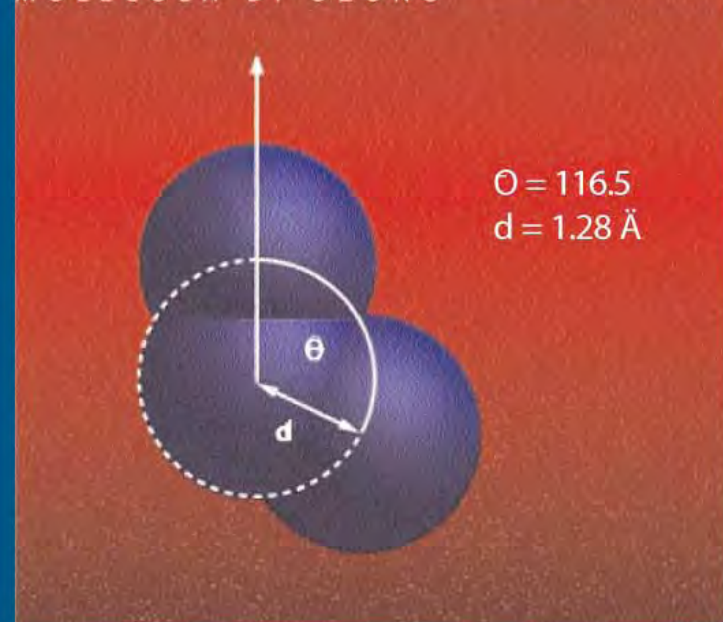
MOLECOLA DI OZONO
