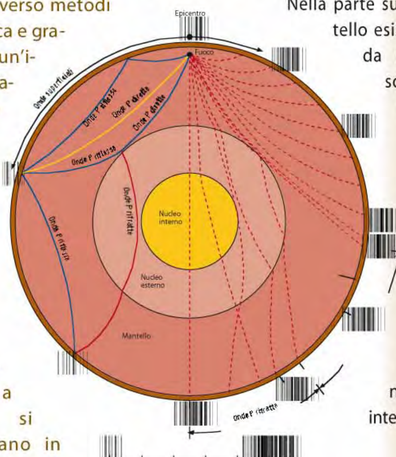
Distribuzione delle onde P generate da terremoto. La riflessione e la rifrazione delle onde P al contatto mantello-nucleo crea una zona d'ombra fra 103 e 143 gradi
