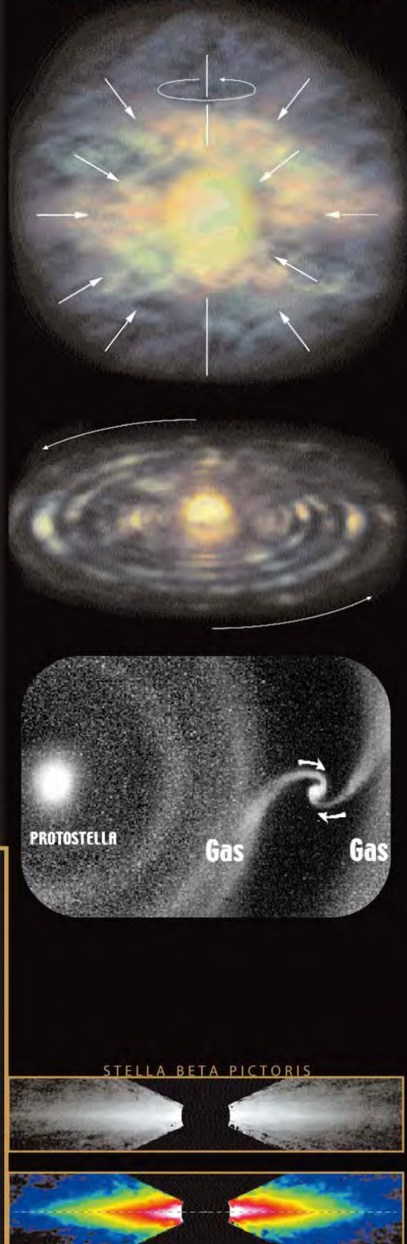
FASI EVOLUTIVE DI UNA COCOON-NEBULA
