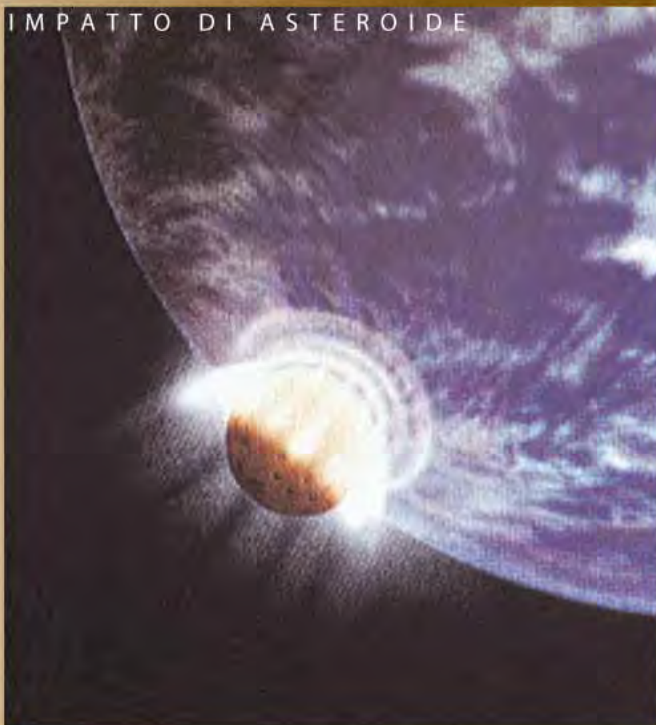
IMPATTO DI ASTEROIDE
