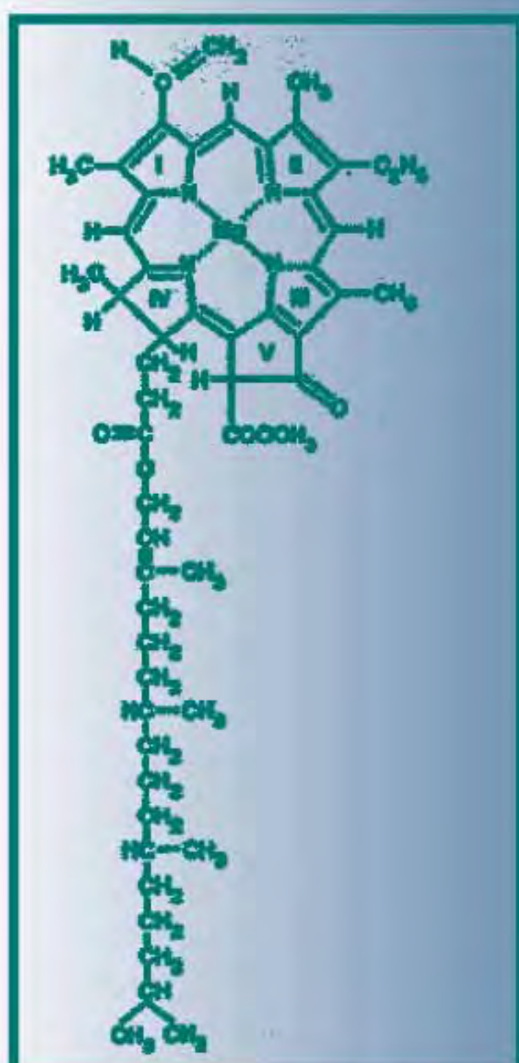
MOLECOLA DELLA CLOROFILLA
